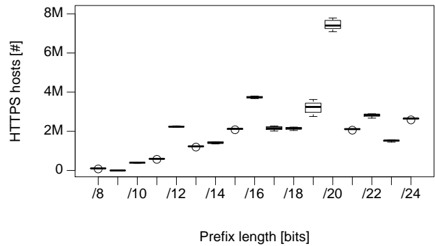
(d) HTTPS for more specific prefixes.
